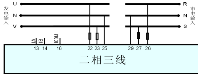
图7 二相三线连接时接线图
