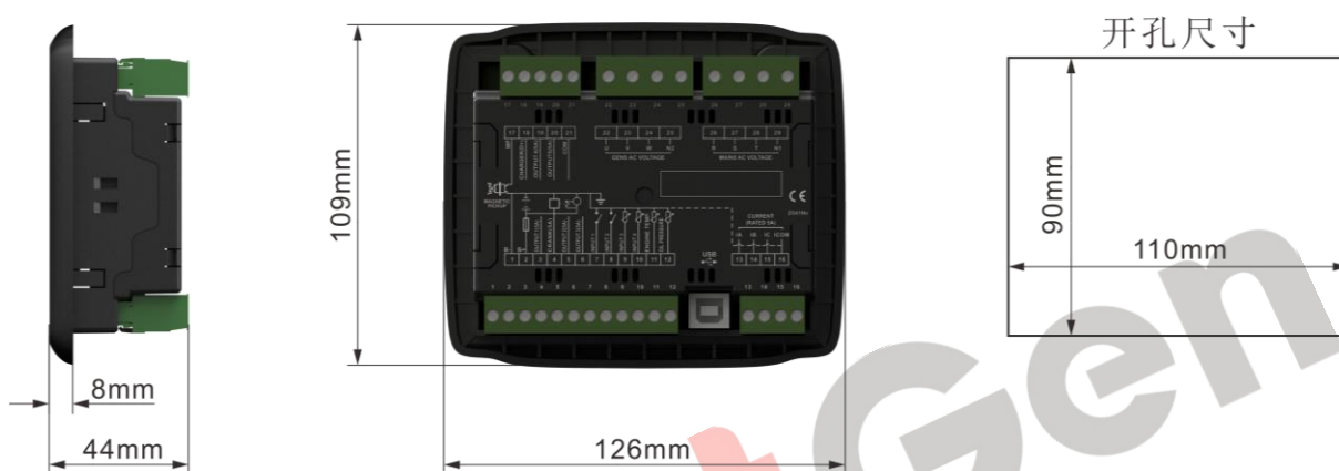
图8 外形及开孔尺寸
