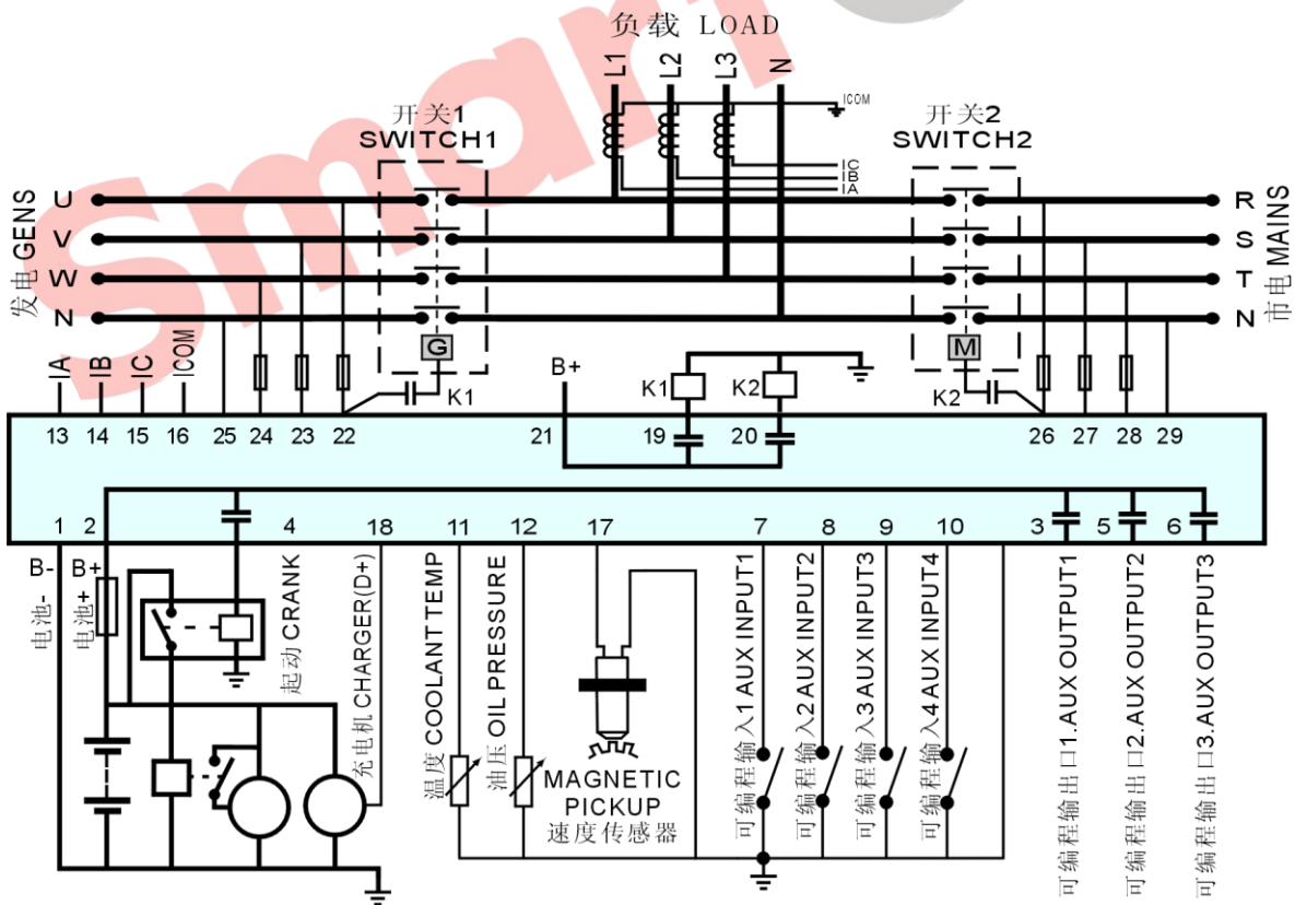
图5 HGM420N 典型应用图
