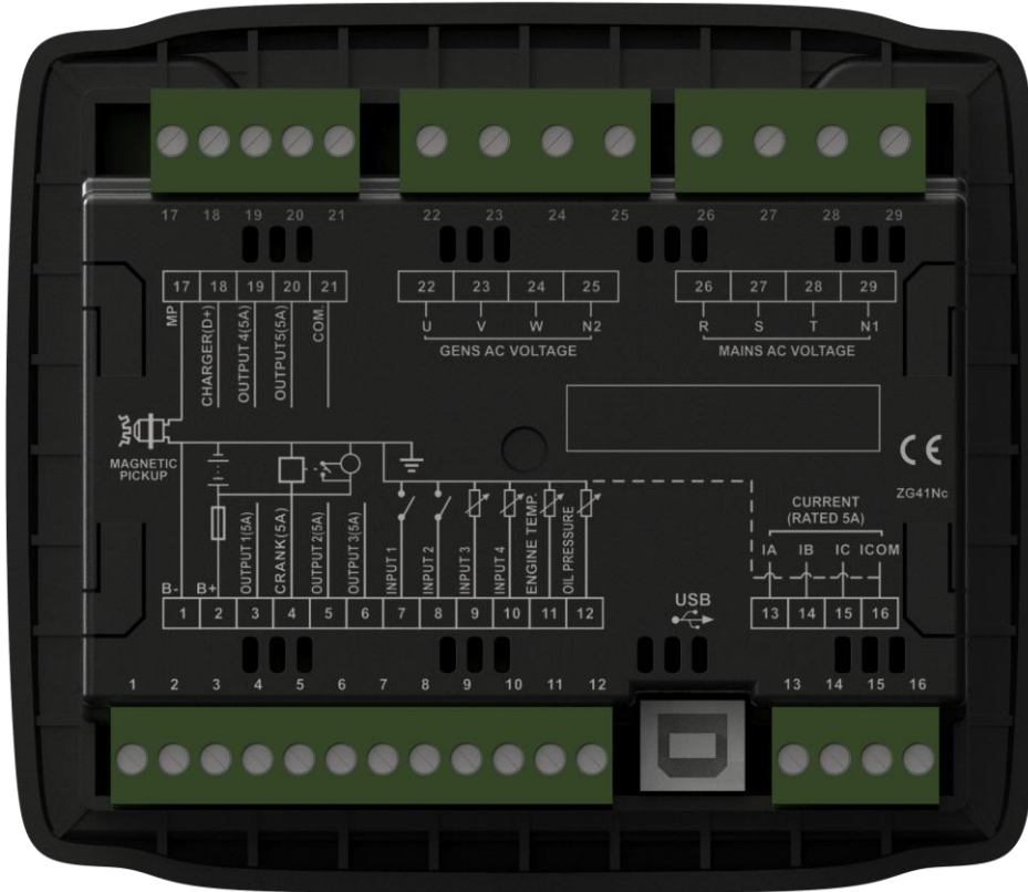
图3 控制器背面板图
