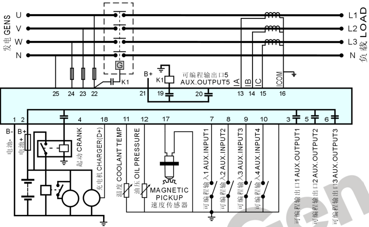
图4 HGM410N 典型应用图
